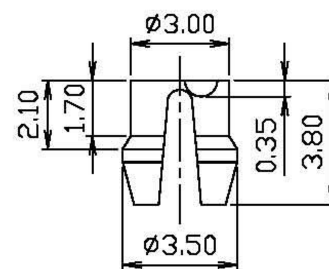
DETAIL Y
