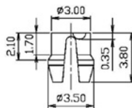
DETAIL Y
