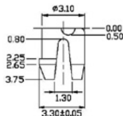
DETAIL Y
