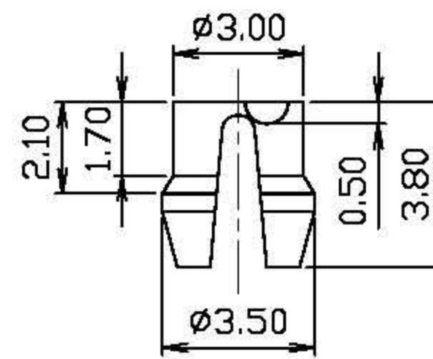
DETAIL Y
