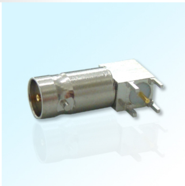
R/A MINI-BNC JACK PCB RECEPTACLE
